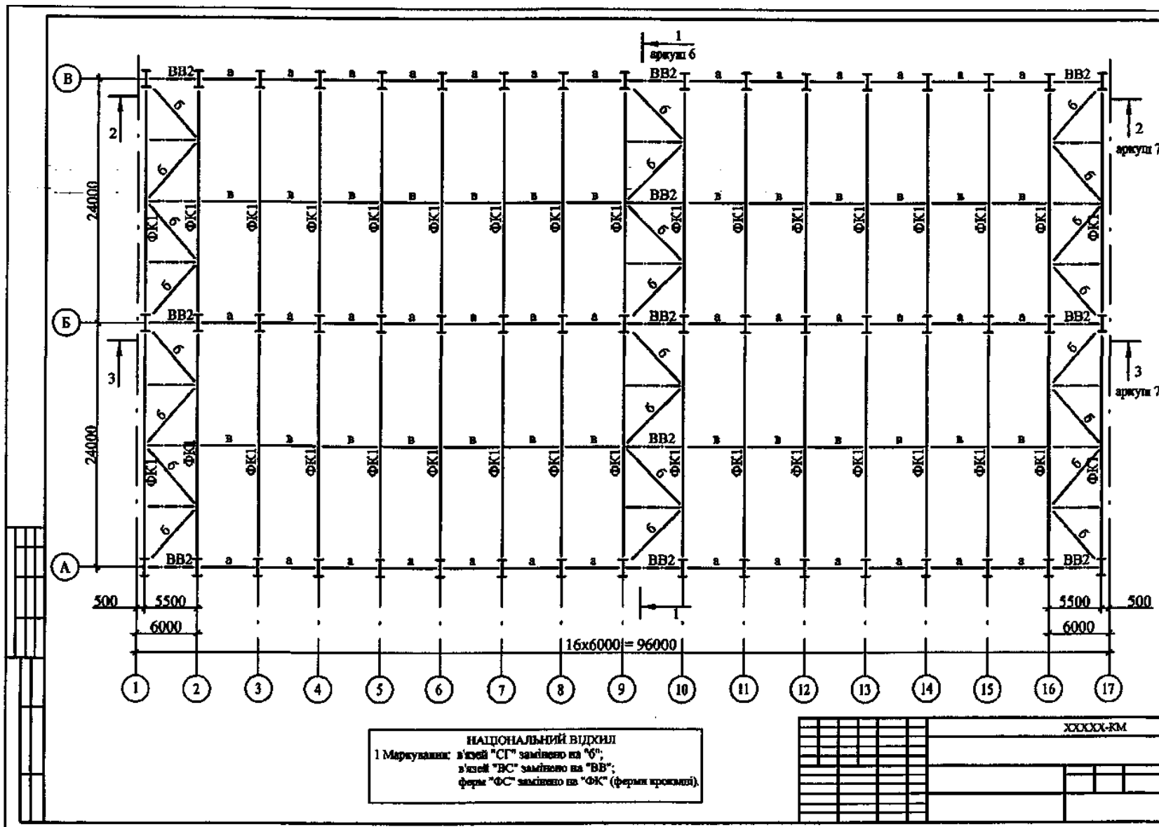
Рисунок Г.2 – Схема розташування елементів покриття по нижніх поясах ферм
