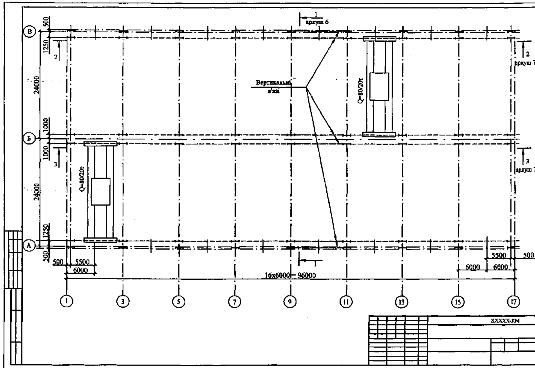
Рисунок Б.4 – Схема розташування колон на відмітці 0,000 м
