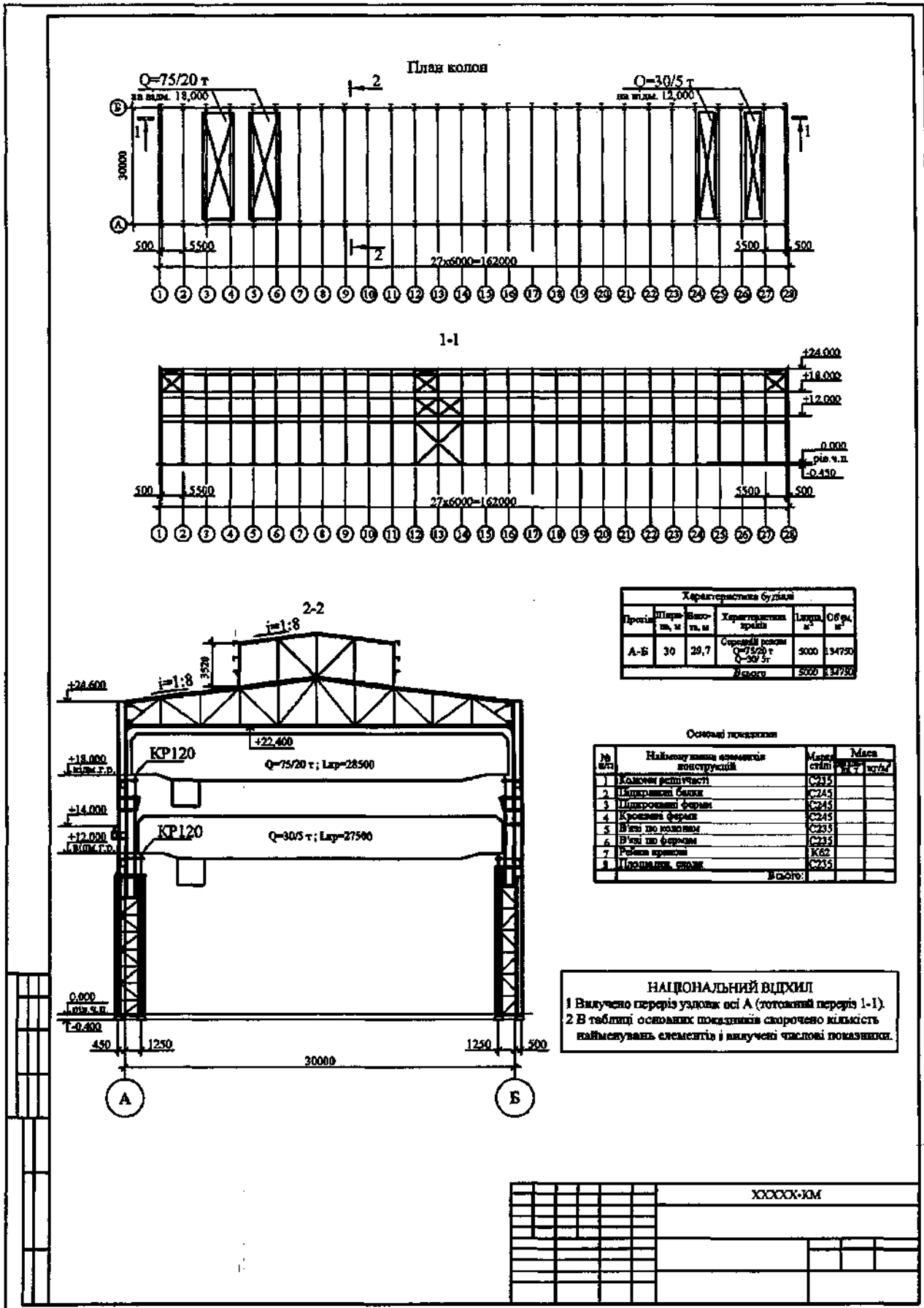
Рисунок Б.3 – Загальний вид
