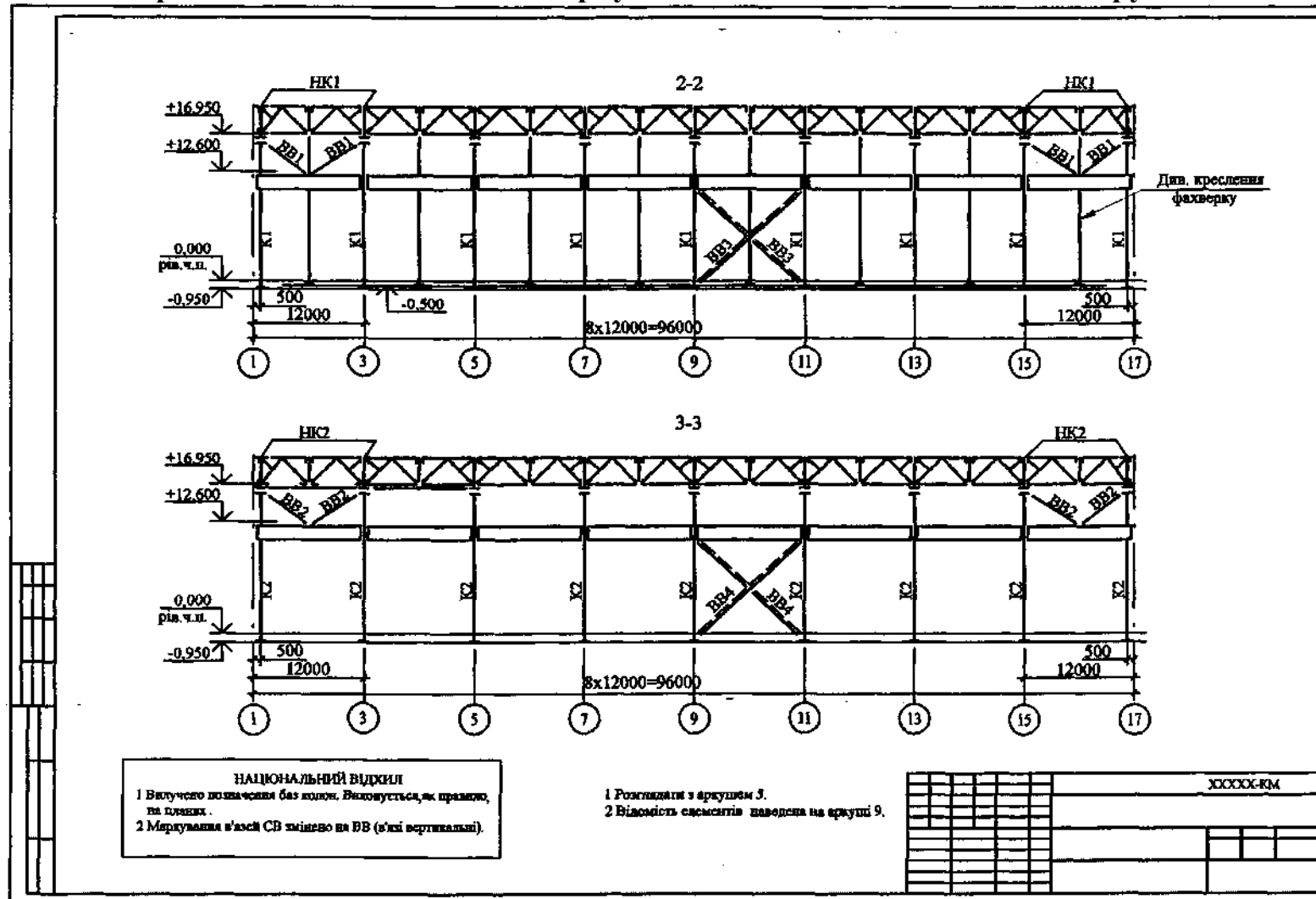
Рисунок Г.1 – Перерізи 2-2; 2-3
