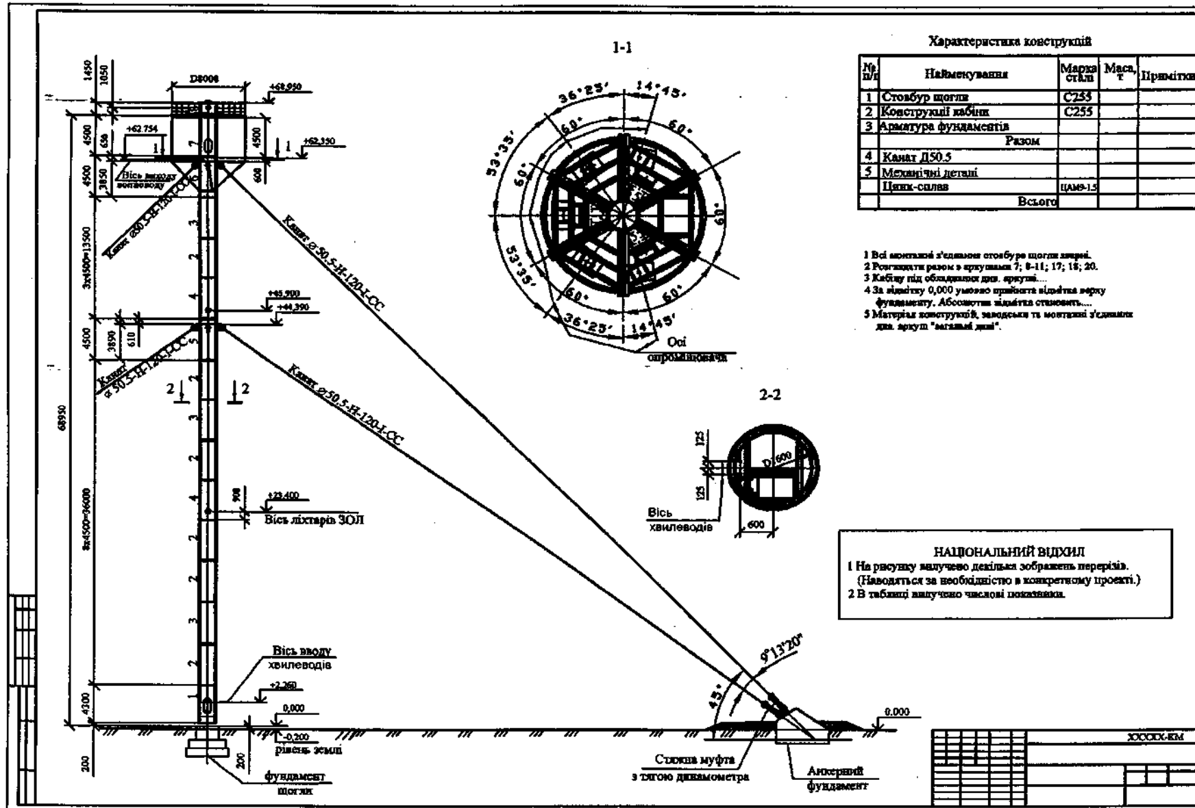
Рисунок Б.2 – Загальний вид щогли
