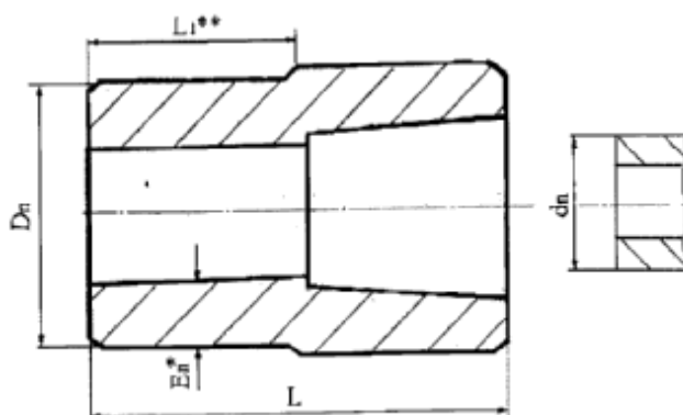
Рисунок 11 - Переход раструбно-цилиндрический
