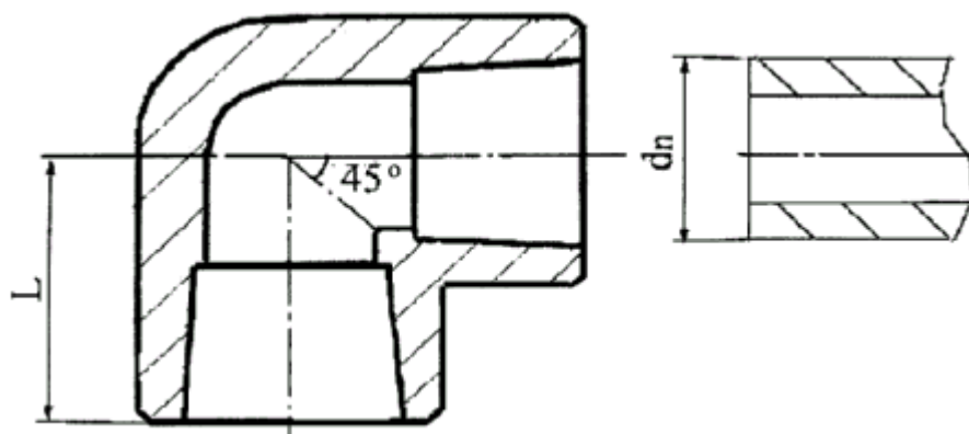
Рисунок 7 - Косинець 90° розтрубний
