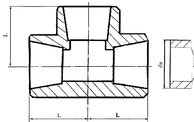
Рисунок 4 - Трійник рівнопрохідний розтрубний
