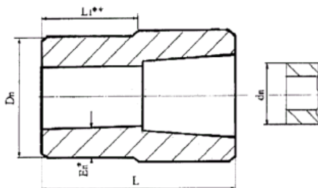
Рисунок 11 - Перехід розтрубно-циліндричний
