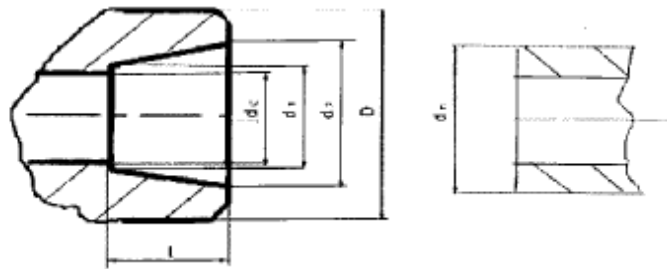
Рисунок 2 - Общая часть соединительной детали для сварки нагретым инструментом в раструб
