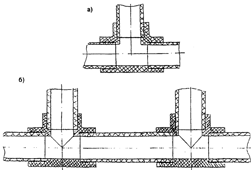
Рисунок Е.1а - Зварювання нагрітим інструментом врозруб трійника рівнопрохідного розтрубного;
