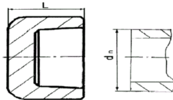
Рисунок 10 - Заглушка розтрубна
