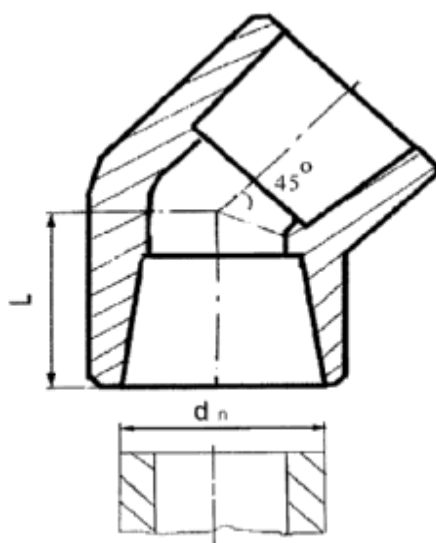
Рисунок 6 - Косинець 45° розтрубний
