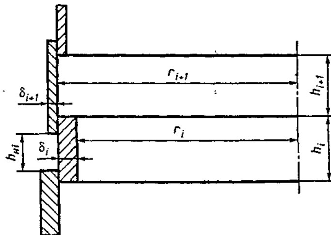
r_i , h_{in} и h_i , \delta_i — внутренний радиус, внешняя и внутренняя высота, толщина стенки i -го пояса соответственно; r_{i+1} , h_{i+1} , \delta_{i+1} — внутренний радиус, внутренняя высота, толщина i + 1 -го пояса соответственно
