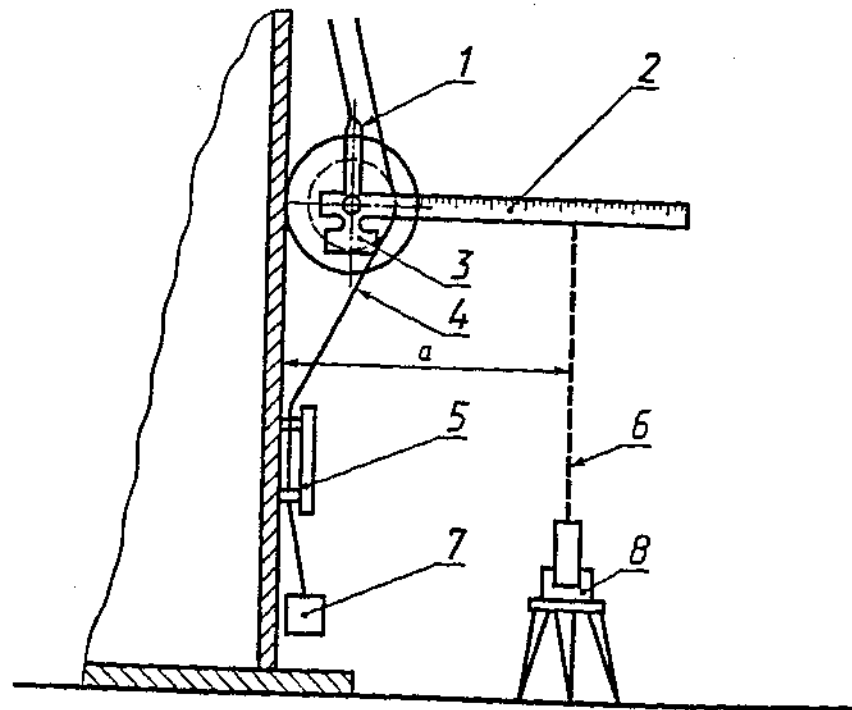
1 — каретка; 2 — линейка; 3 — противовес; 4 — струна; 5 — магнитный держатель; 6 — визирная линия; 7 — груз; 8 — теодолит; a — расстояние от стенки резервуара до нити отвеса Рисунок А.4 — Схема измерения радиальных отклонений с применением измерительной каретки с теодолитом
