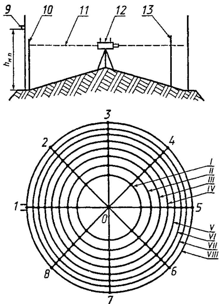
1—8 — радиусы, 9 — приемно-раздаточный патрубок, 10 — рейка; 11 — горизонт нивелира; 12 — нивелир; 13 — рейка в точке касания дна грузом рулетки, I—VIII — концентрические окружности, h_{мп} — высота «мертвой» полости резервуара
