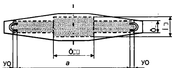
Рисунок 2 — Утримувальний ремінь з інтегрованими з'єднувальними засобами для ремня. Головні складові частини
