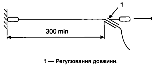
Рисунок 6 — Випробовування статичної стійкості до навантажень з'єднувальних засобів утримувального ременя
