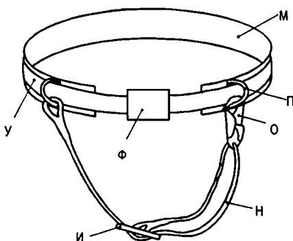
Рисунок 2 — Утримувальний ремінь з інтегрованими з'єднувальними засобами для ремня. Головні складові частини
