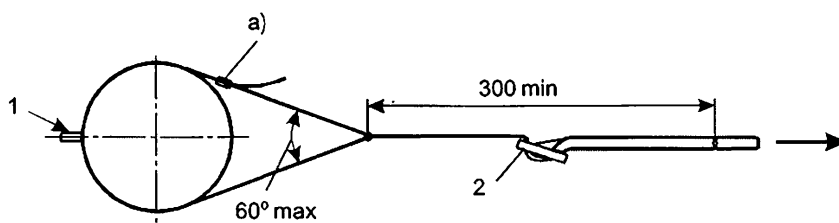
Рисунок 4 — Випробовування статичної стійкості до навантажень утримувального ременя
