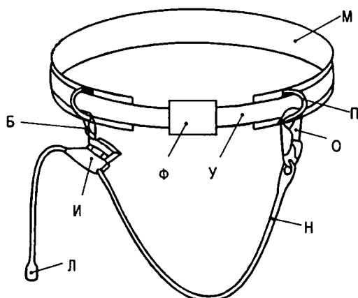
Рисунок 1 — Утримувальний ремінь із з'єднувальними елементами, які закріплені двома петлями
