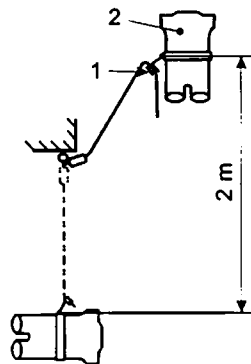
Рисунок 6 — Випробовування статичної стійкості до навантажень з'єднувальних засобів утримувального ременя
