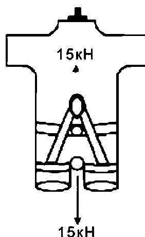
Рисунок 5 — Випробовування статичної сили спорядження для роботи сидячи
