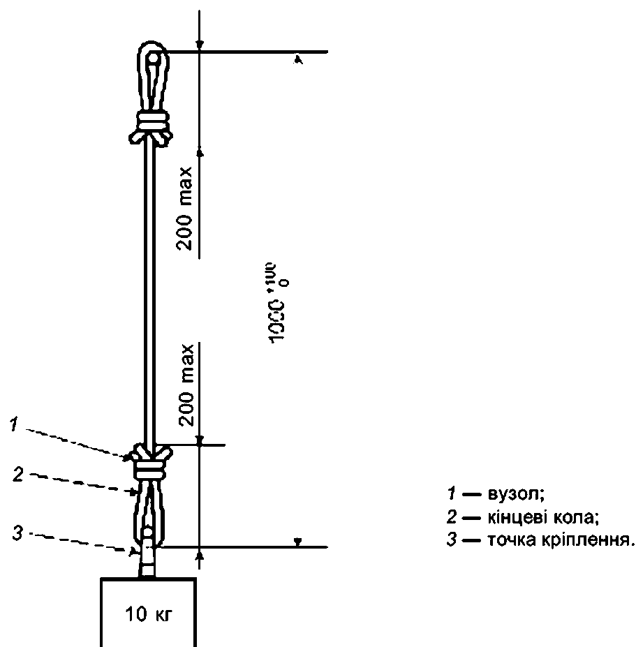
Рисунок 3 — Строп для випробовування динамічних характеристик
