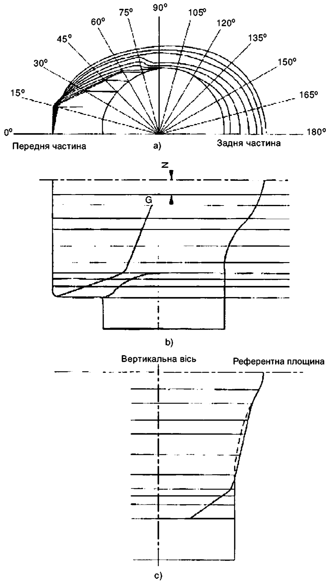
Рисунок 3 — Основні дані макета голови нижче референтної площини
