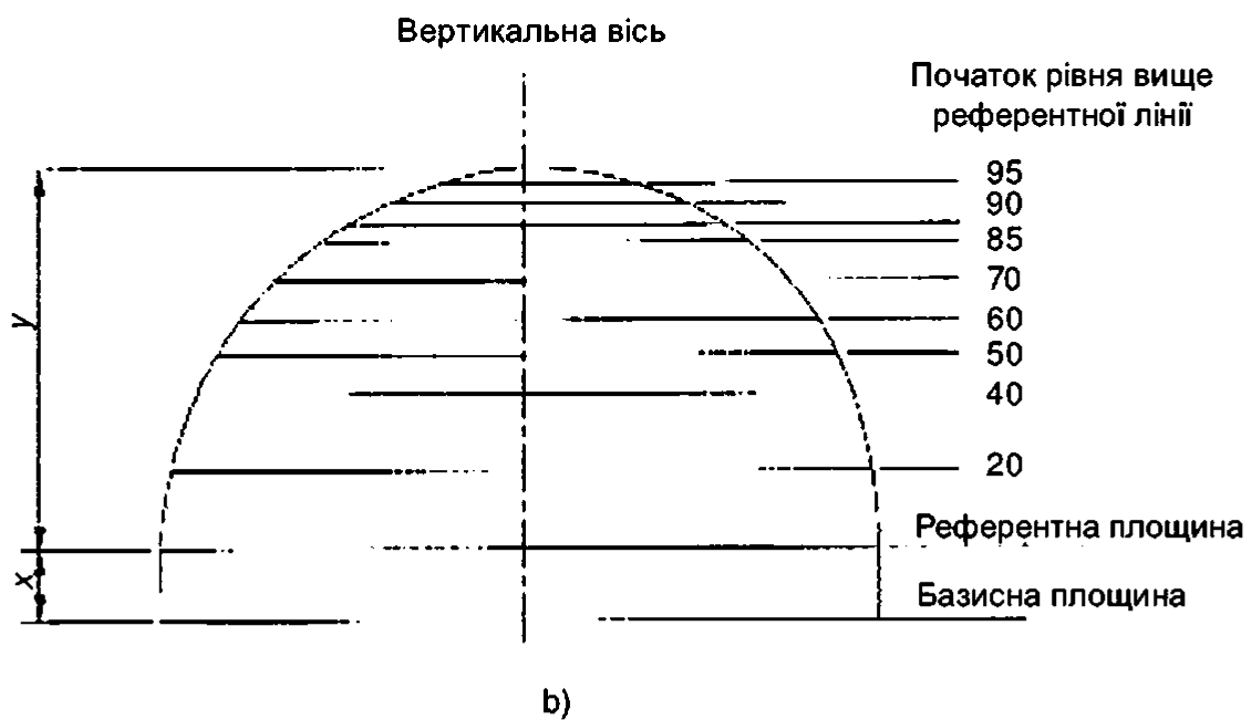
Рисунок 2 — Нормальний макет голови вище базисної площини
