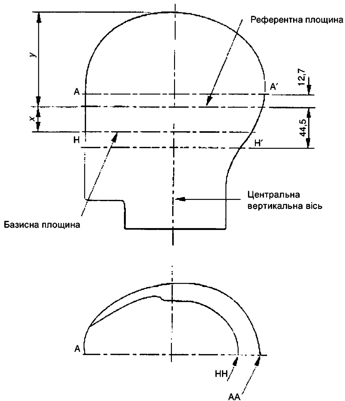
Рисунок 1 — Головні площини макета голови
