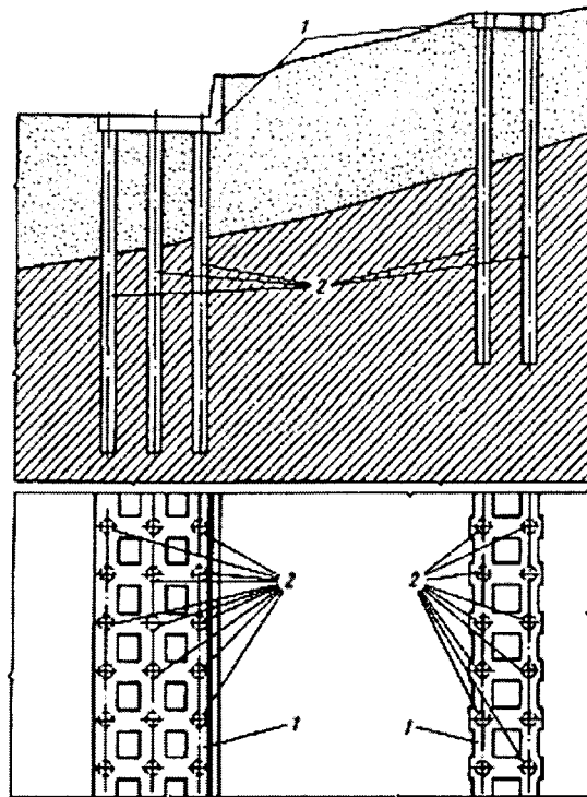
Рисунок 6.19 – Утримуюча протизсувна споруда з двох окремих палиових стрічок
