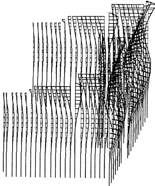
Рисунок Б.2.4 – Розрахункова схема утримуючої споруди. Перетин. Розподіл згинальних моментів M_z (тм) в елементах паль утримуючих схил конструкцій
