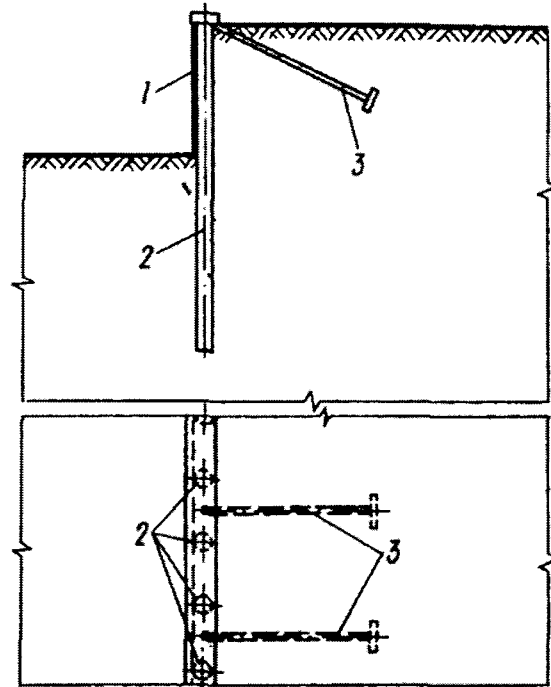
1 – залізобетонна закидка; 2 – палі; 3 – анкери
