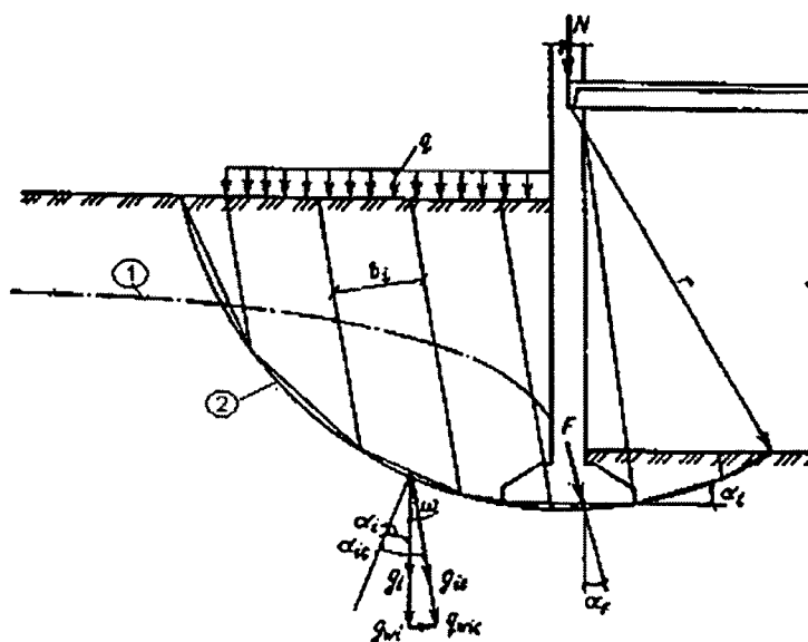
Рисунок 8.20 – Розрахункова схема для визначення стійкості стіни підвалу проти зрушення по круглоциліндричних поверхнях
