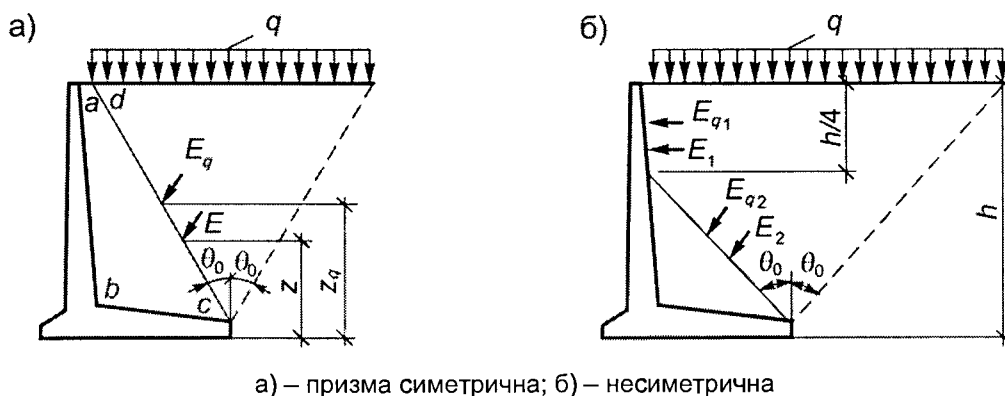
Рисунок 7.10 – Схеми до визначення активного тиску ґрунту на кутникові підпирні стіни з різними призмами обвалення.
