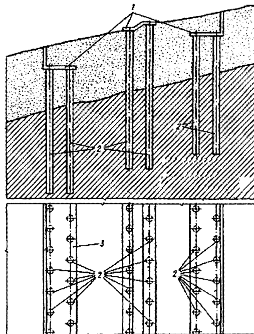
Рисунок 6.18 – Утримуючі протизсувні споруди з трьох окремих палевих стрічок
