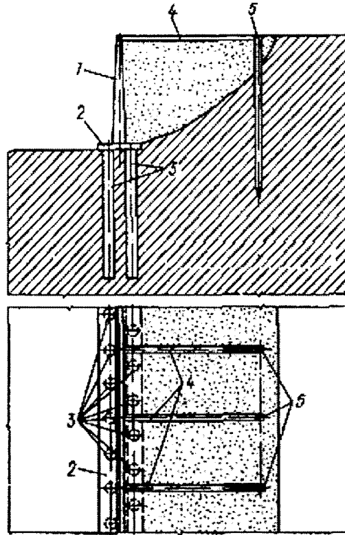
Рисунок 6.7 – Підпірна стіна, що зводиться на дворядних бурових палях, об'єднаних ростверком
