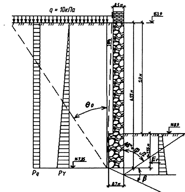
Рисунок Б 1.2 – Схема до розрахунку підпірної стіни
