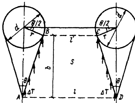
Рисунок 8.13 – Схема до розрахунку відстані між палями при однорядній пальовій огорожувальній конструкції
