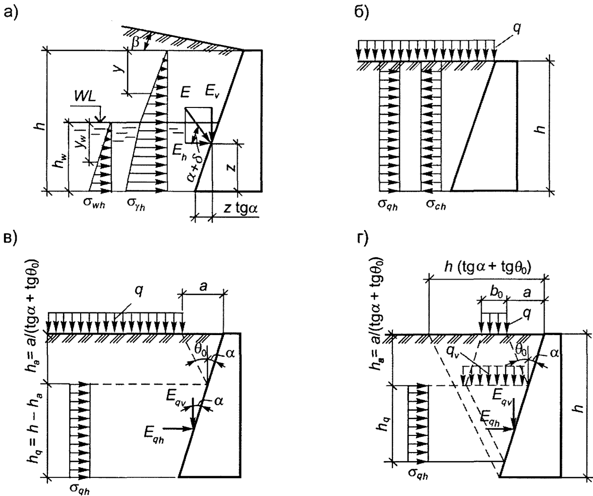
а – від власної ваги і тиску ґрунту; б – від рівномірно-розподіленого навантаження; в – від фіксованого навантаження; г – від смугового навантаження
