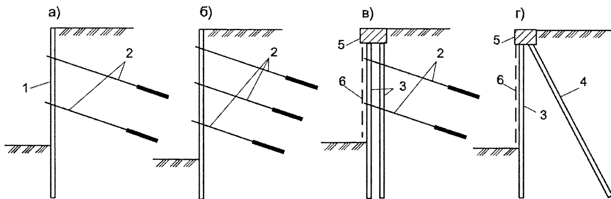
а, б – стіни шпунтові, пальові чи траншейні з анкерами (тимчасові); в – стіни пальові багаторядні з анкерами (тимчасові); г – стіни у вигляді козлових пальових систем (постійні) 1 – стіни; 2 – анкери; 3 – палі вертикальні; 4 – палі нахилені; 5 – ростверки; 6 – екрани
