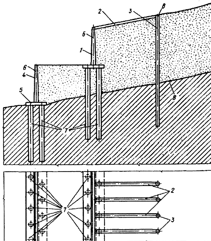
Рисунок 6.19 – Утримуюча протизсувна споруда з двох окремих палиових стрічок
