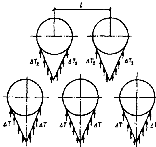
Рисунок 8.14 – Схема розрахунку багаторядної пальової огорожувальної конструкції
