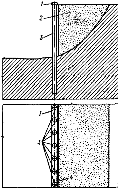
Рисунок 6.5 – Однорядна підпірна стіна з бурових палей, об'єднаних ростверком
