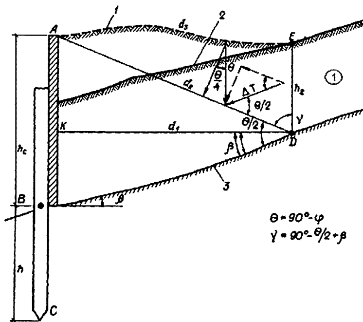
Рисунок 8.19 – Схема до розрахунку висоти утримуючої панельної стіни на зсувах
