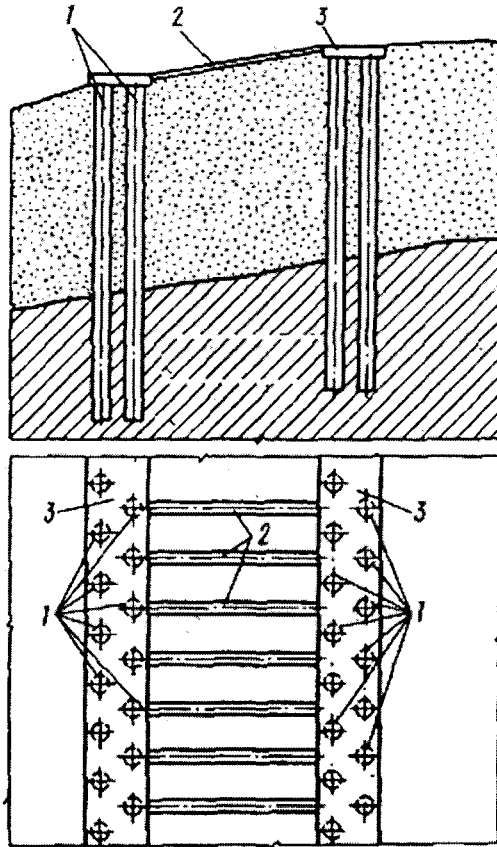
Рисунок 6.13 – Дворярусна пальова огорожувальна конструкція з дворядних бурових палей, об'єднаних ростверками і зв'язками
