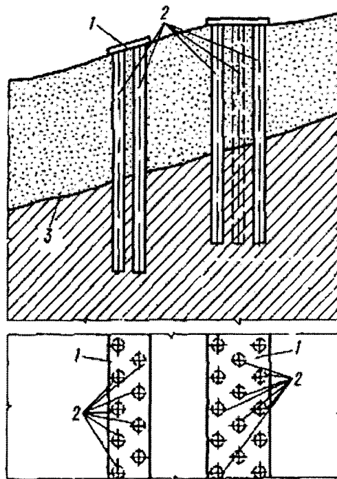
Рисунок 6.14 – Дворярусна пальова огорожувальна конструкція без зв'язок
