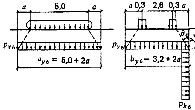
Рисунок 7.8 – Схема тиску від гусеничного навантаження НГ-60 при русі вздовж споруди
