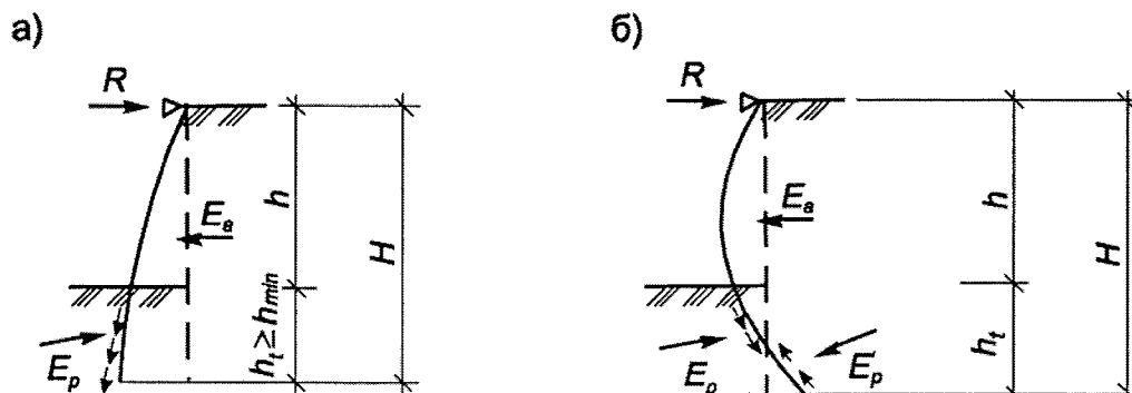
а – жорстка стіна; б – гнучка стіна
