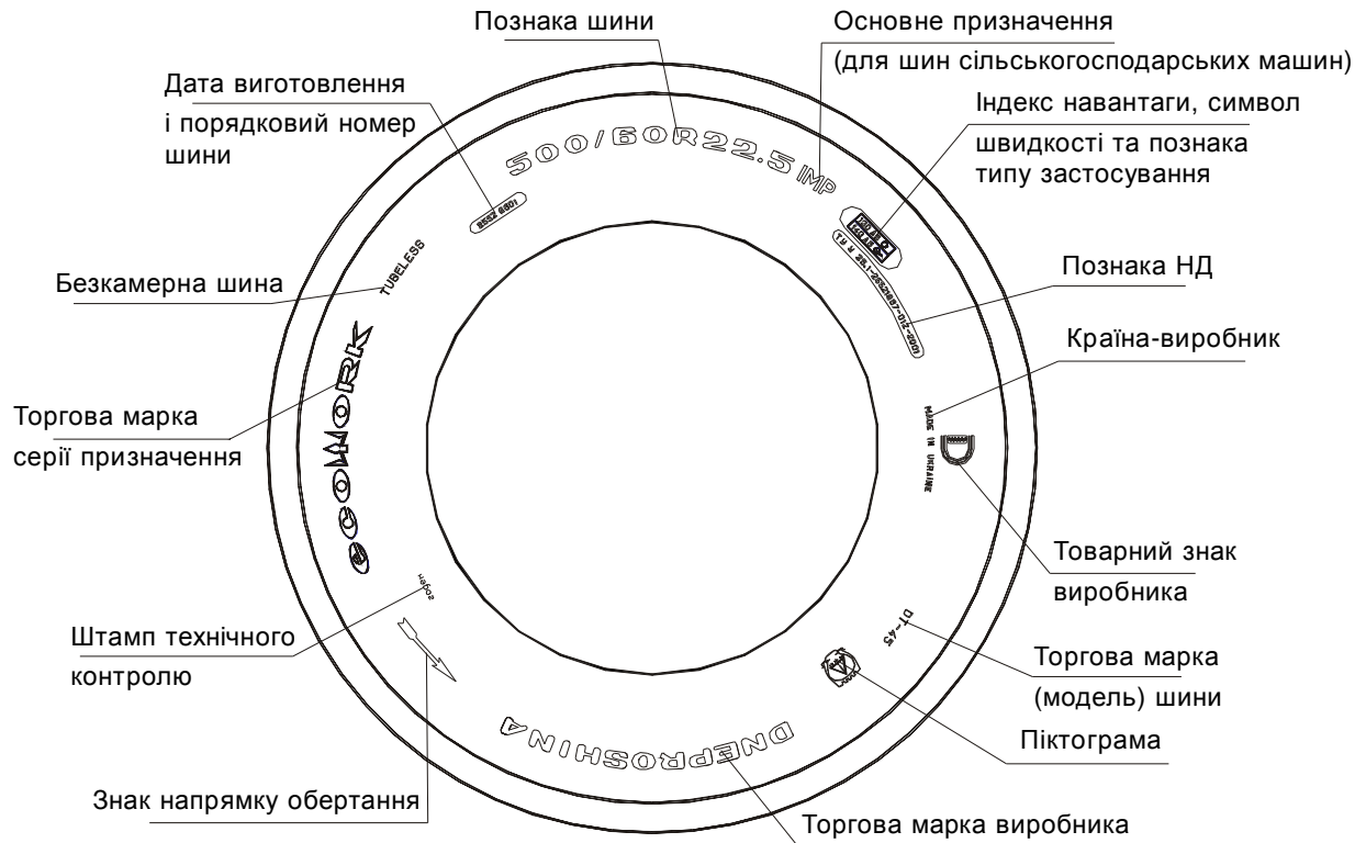
Рисунок 1 — Схема розташування маркування на пневматичній шині
