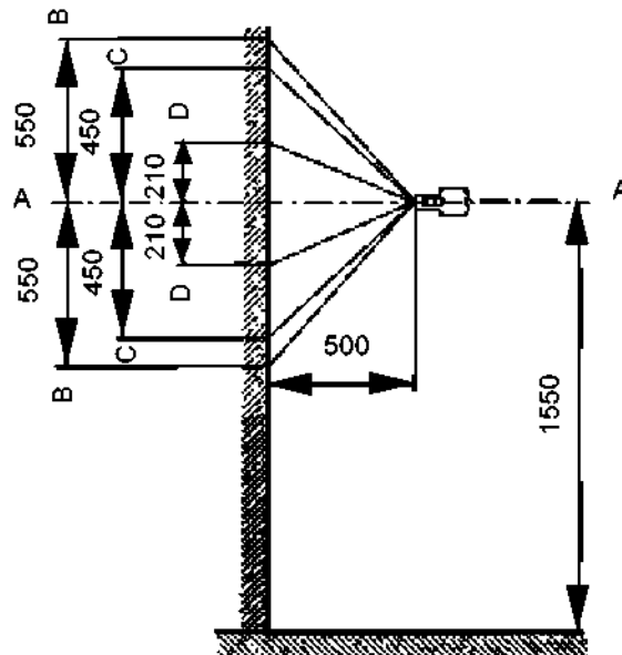
Рисунок Е.2 - Схема розташування обладдя під час випробовування з визначання кута розпилювання
