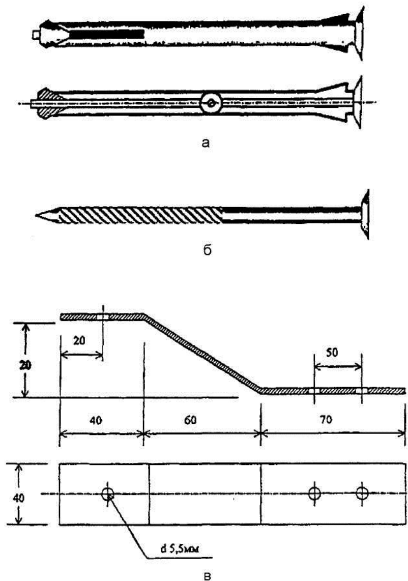
Рисунок Б.1 - Приклади конструкції кріпильних елементів
