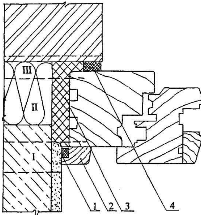
Рисунок А.4 - Вузол бічного примикання дерев'яного блока до стінового прорізу з чвертю
