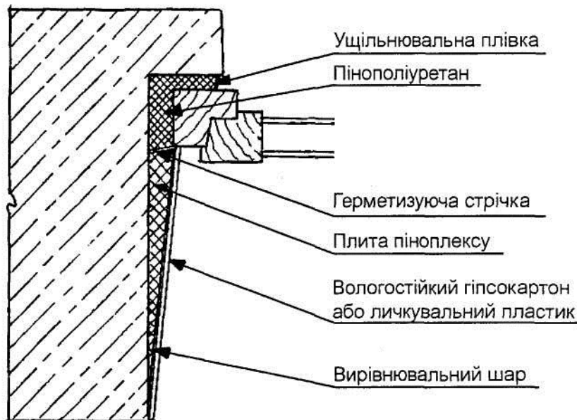
Рисунок 5 - Схема конструкції вузла примикання блока до стінового прорізу з утепленням внутрішніх укосів
