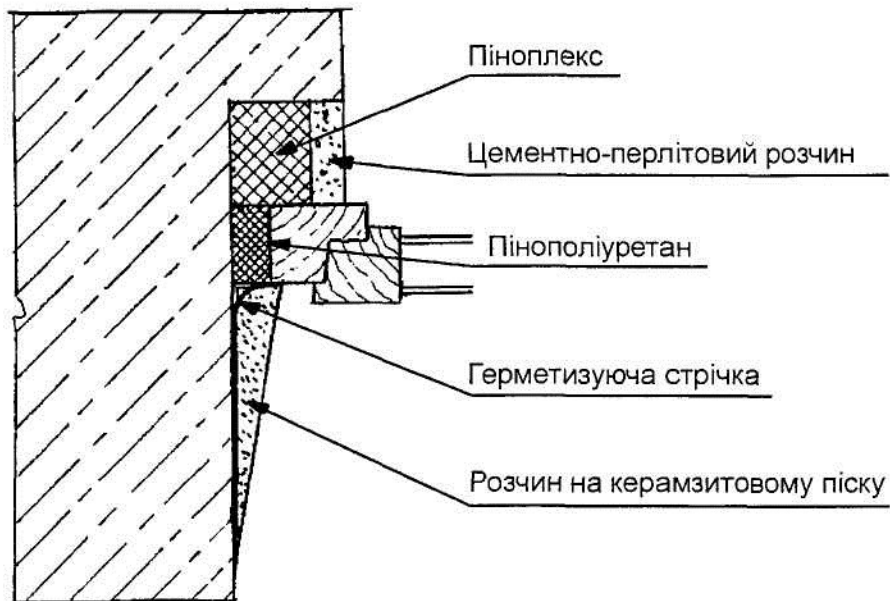
Рисунок 6 - Схема конструкції вузла примикання блока до стінового прорізу з утепленням зовнішніх і внутрішніх укосів
