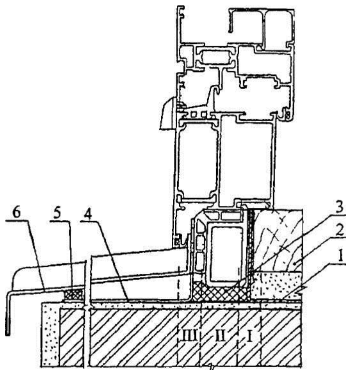
Рисунок А.6 - Вузол бічного примикання блока з алюмінієвих профілів до стінового прорізу з чвертю
