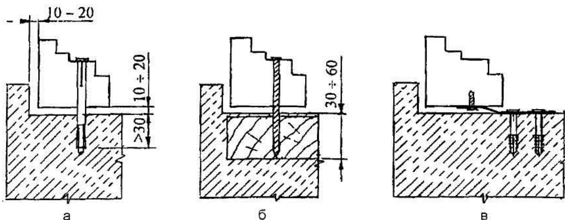
Рисунок Б.2 - Приклади схем кріплення блоків до стіни
