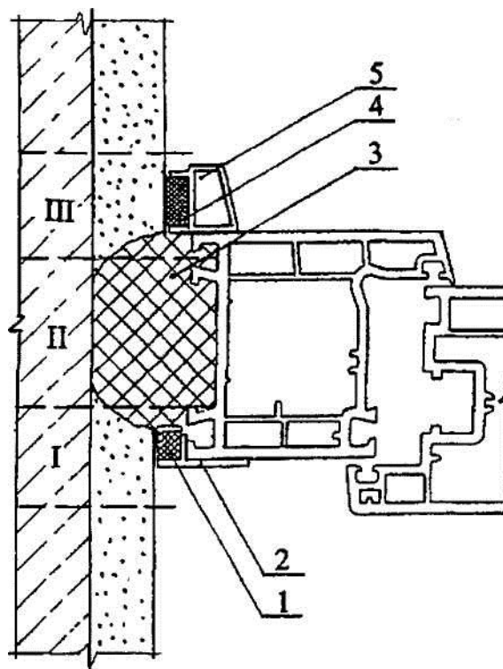
Рисунок А.2 - Вузол бічного примикання блока з ПВХ профілів до стінового прорізу з чвертю
