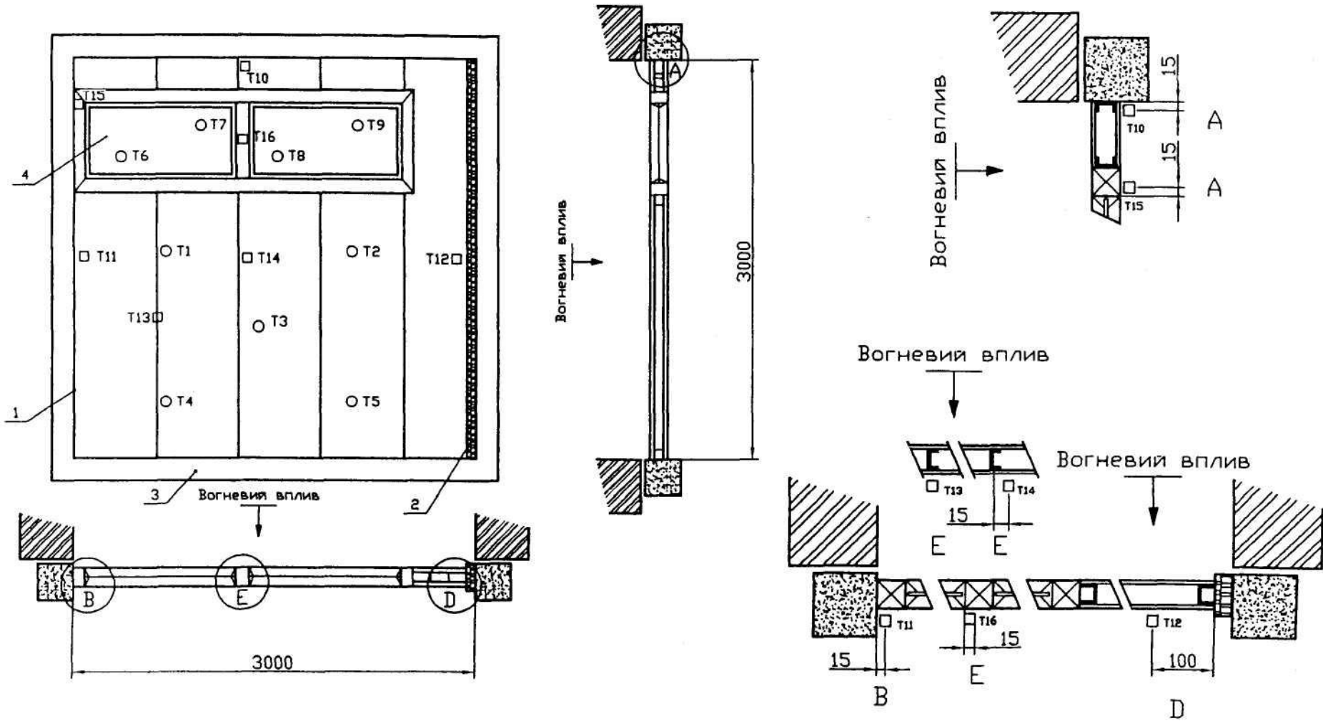
1 - закріплений край зразка; 2 - ущільнення між незакріпленим краєм зразка і опорною конструкцією; 3 - опорна конструкція; 4 - скління; T1-T5 - термопари на необігрівній поверхні зразка для вимірювання середньої температури; T6-T9 - термопари на необігрівній поверхні зразка для вимірювання середньої температури на ділянці зі склінням; T10-T14 - термопари на необігрівній поверхні зразка для вимірювання максимальної температури; T15-T16 - термопари на необігрівній поверхні зразка для вимірювання максимальної температури на зразку із засклінням
