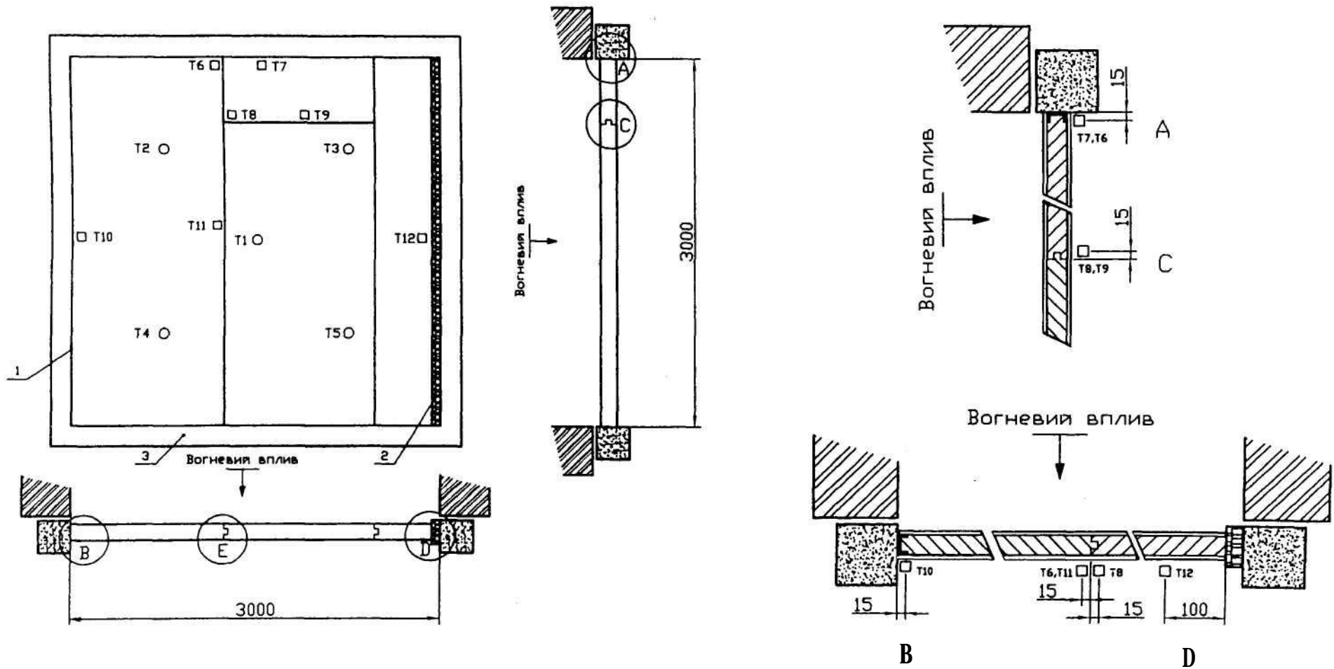
1 - закріплений край зразка; 2 - ущільнення між незакріпленим краєм зразка та опорною конструкцією; 3 - опорна конструкція; T1-T5 - термомпари на необігрівній поверхні зразка для вимірювання середньої температури; T6-T12-термомпари на необігрівній поверхні зразка для вимірювання максимальної температури
