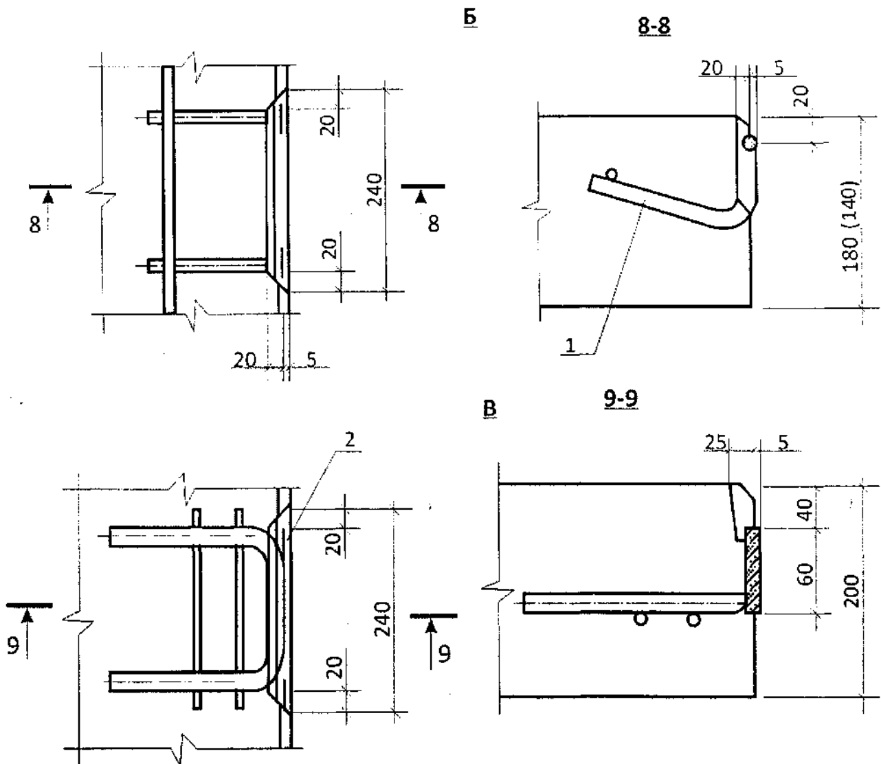
В скобках указан размер для плиты ПАГ-14 1 – стыковое изделие М2 или М4; 2 – стыковое изделие М4а
