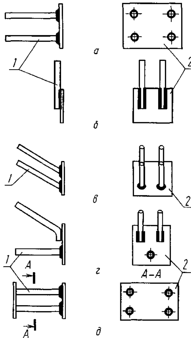
а, б, в, г – закладные изделия открытого типа (соответственно с перпендикулярным, параллельным, наклонным и смешанным расположением анкерных стержней); д – закладное изделие закрытого типа (с перпендикулярным расположением анкерных стержней); 1 – анкерные стержни; 2 – плоский элемент
